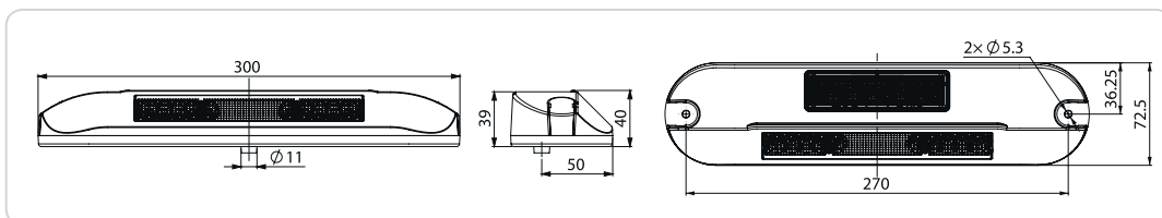
Lampa na wysokości 2,5 m Lamp at 2,5 m height
